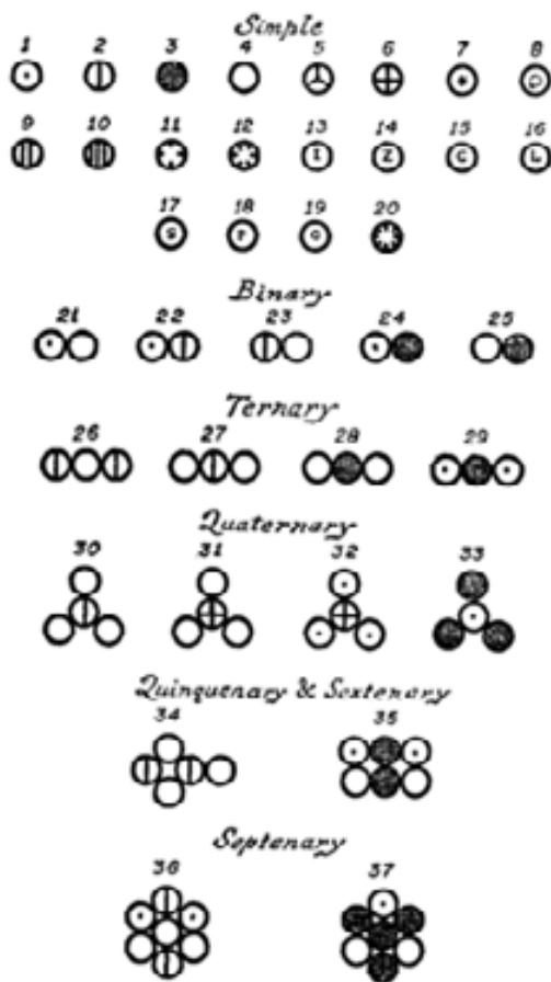
Figura 21. Símbolos dados por Dalton a algúns elementos e compostos. Entre eles, hidróxeno (1), xofre (2), carbo- no (3), osíxeno (4), nitróxeno (6), cobre (15), prata (17), ouro (19) e auga (21). Equivocouse coa auga, describindoa como HO en lugar de H 2 O, pero as súas fórmulas para o monóxido de carbono (25) e dióxido de carbono (28) eran correctas.
