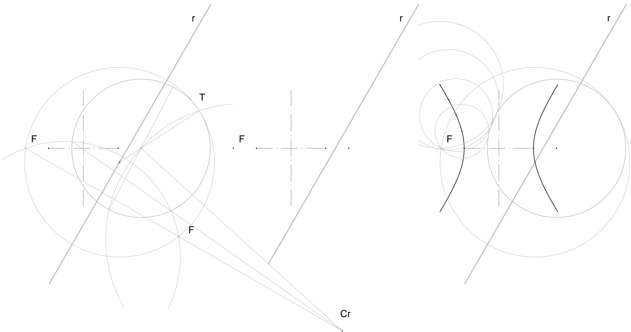
Hiperbole: Lugar geometrico de los centros de circunferencia tangentes a la circunferencia focal de un foco y que pasan por el otro,
