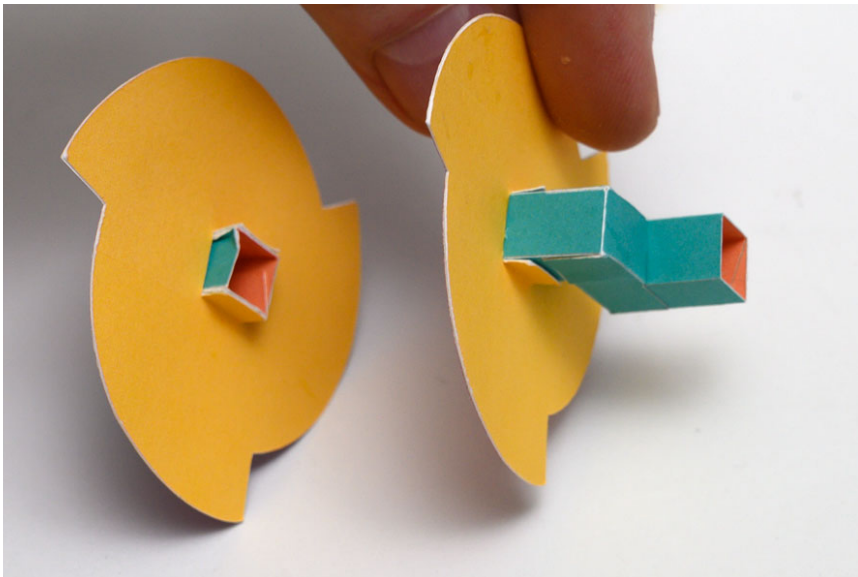
6. Pega dúas levas aliñadas, encaixa as bielas no seu sitio.
