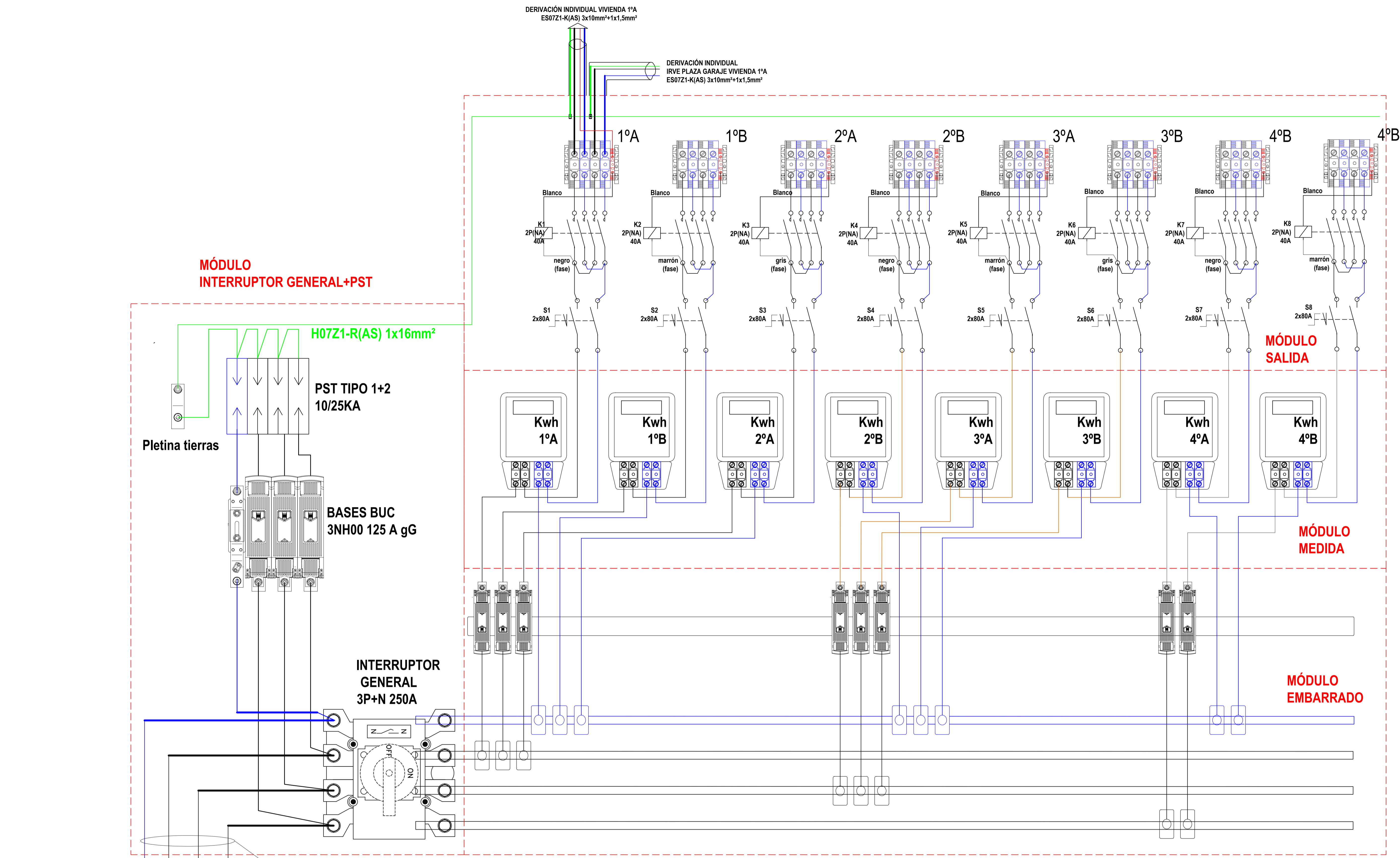
ESQUEMA DE CENTRALIZACIÓN PARA 8 SUMINISTROS MONOFÁSICOS CON IRVE INDIVIDUAL VÁLIDO PARA ESQUEMAS 2 3A 3B y 4A DE LA ITC-BT-52 DEL REBT
