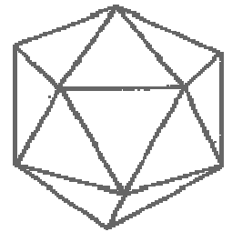
Icosaedro
