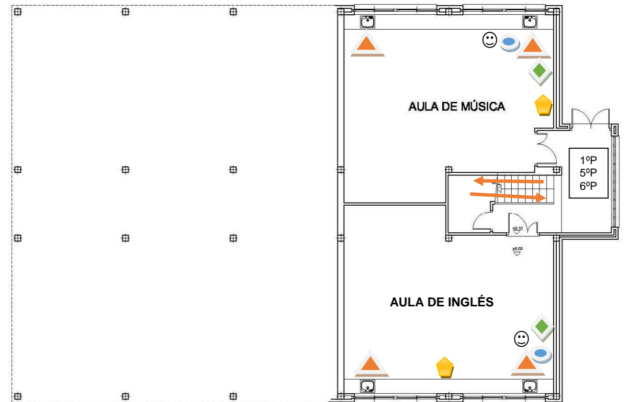
PLANTA DE S/S
