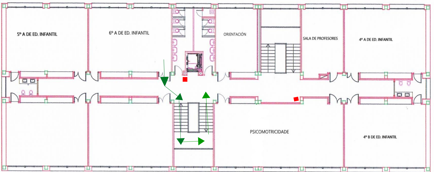
PLANTA PRIMEIRA
