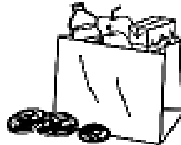
La compra
